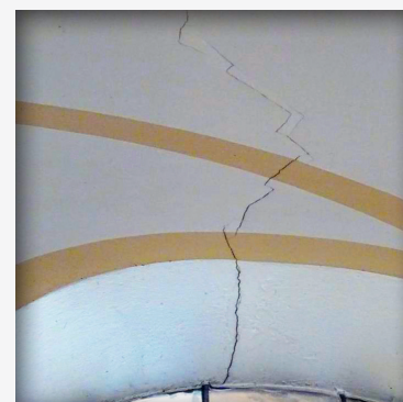
Risse im Mauerwerk
